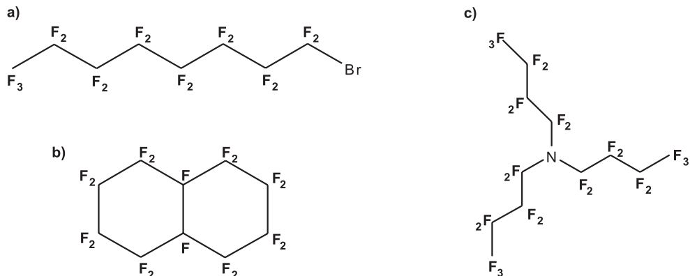
Rys. 1. Struktury chemiczne przykładowych cząsteczek perfluorozwiązków: a) bromku perfluorooktylu (PFC alifatyczny), b) perfluorodekalina (PFC cykliczny) oraz c) perfluorotributyloaminy (perfluorowana pochodna aminy organicznej).
