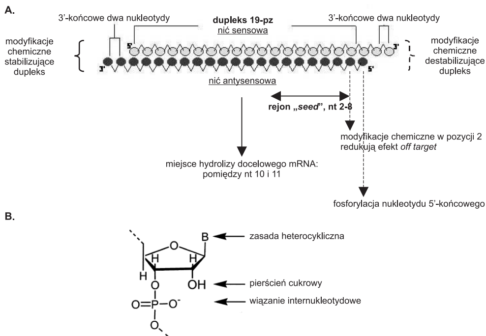
Rys. 1. A. Struktura dupletu siRNA, B. miejsca w nukleotydzie odpowiednie do wprowadzania modyfikacji chemicznych.
